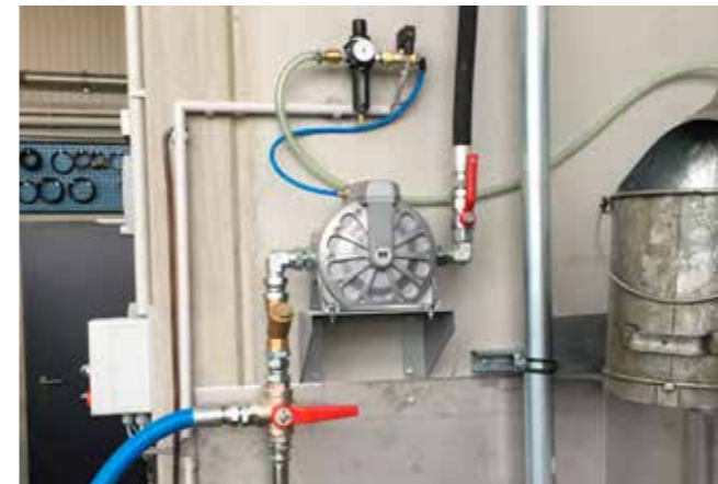
Die fest installierte Druckluft-Membranpumpe DF 50 pumpt in Hamburg das Altöl in den dafür bereitstehenden Tank
